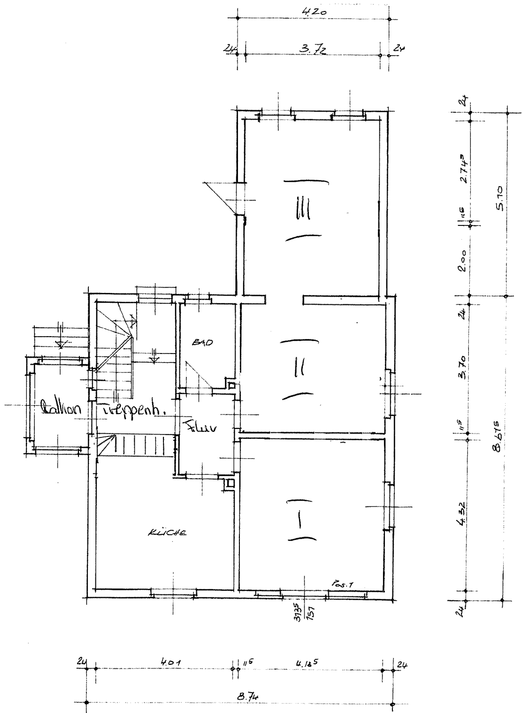
DACH GESCHOSS
