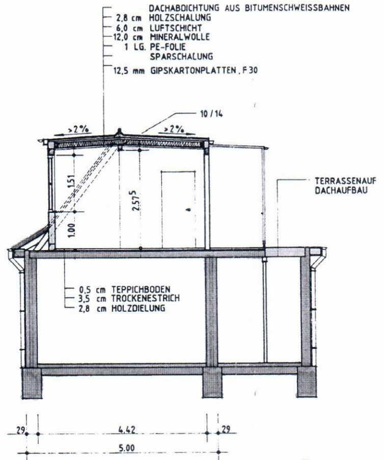
SNITT B-B
