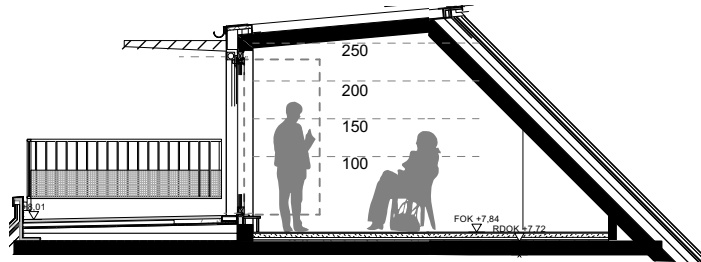
Schnitt
