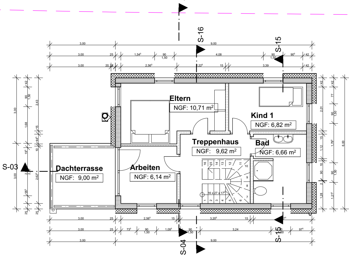
Grundriss Obergeschoss
