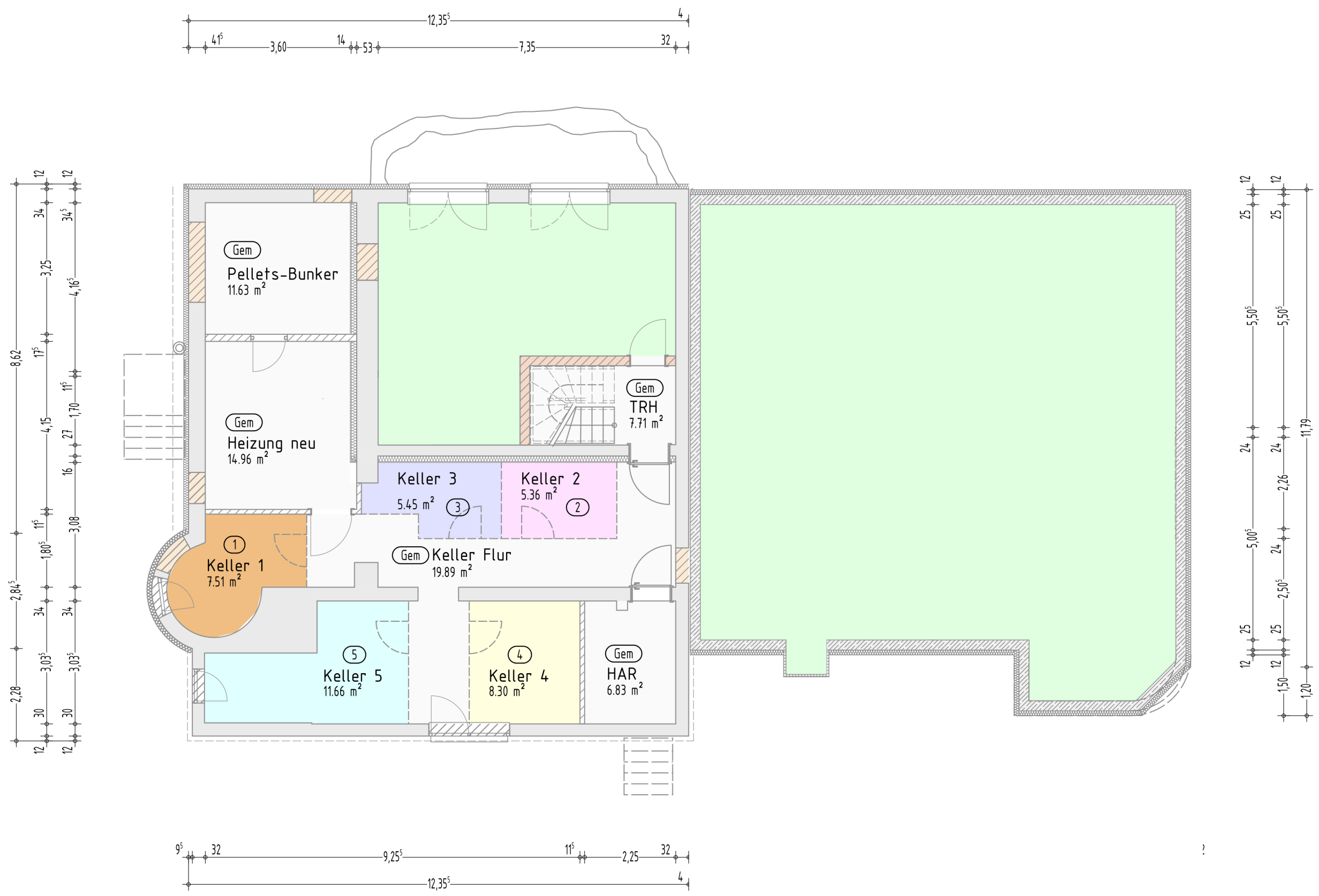
GRUNDRISS KELLERGEBOSS
