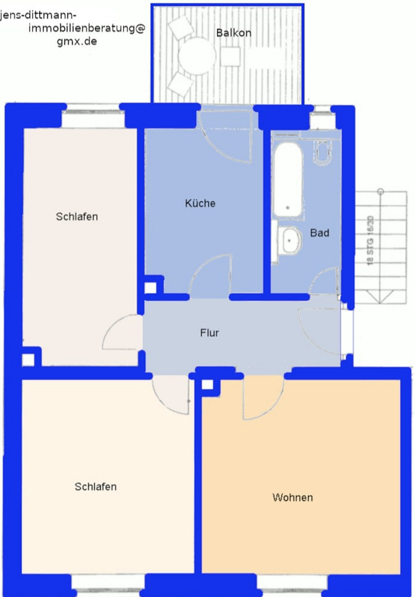
Grundriss 3R 1.OG
