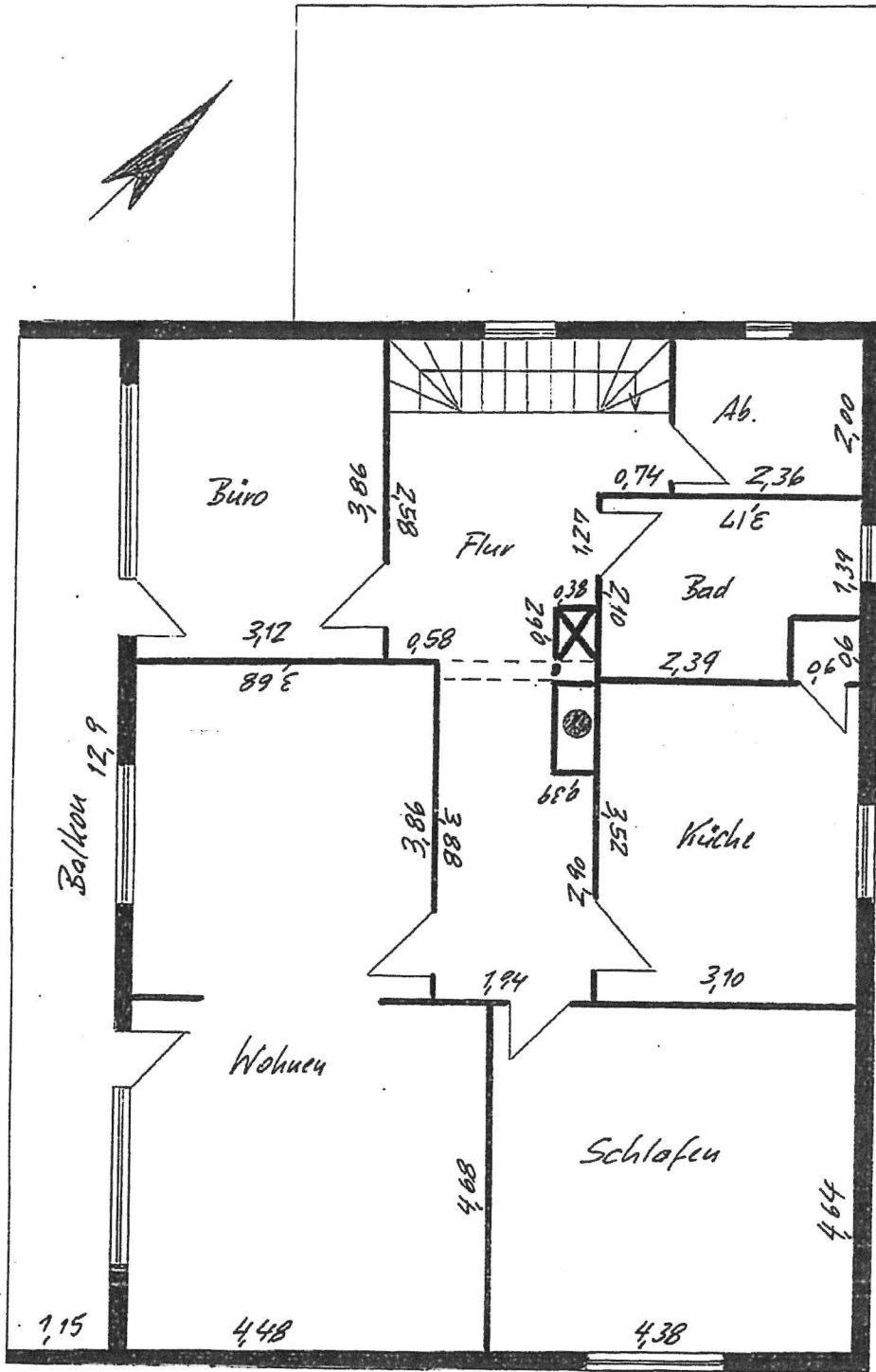
(Obergeschossgrundriss – ohne Maßstab)
