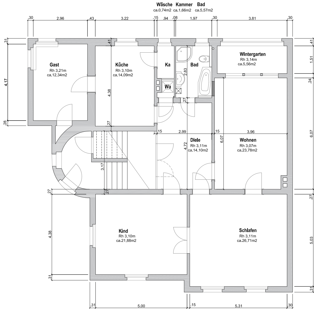
Grundriss Schillerstr. 1 EG
