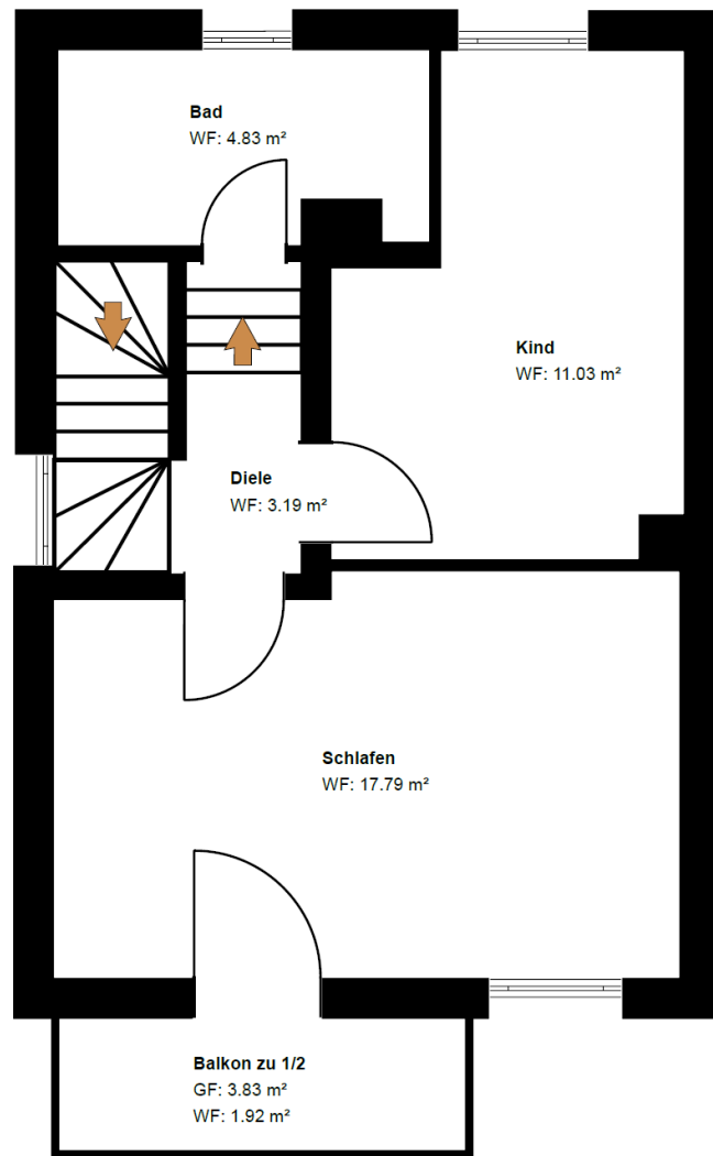
Obergeschoss
