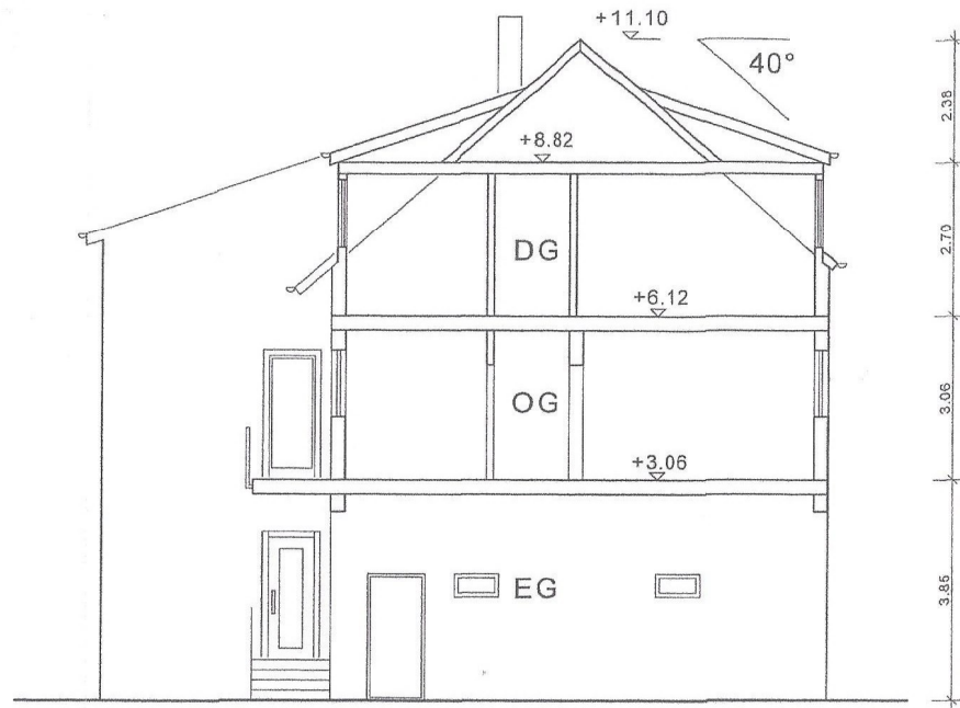
SCHNITT B-B
