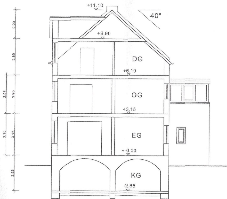
SCHNITT A-A
