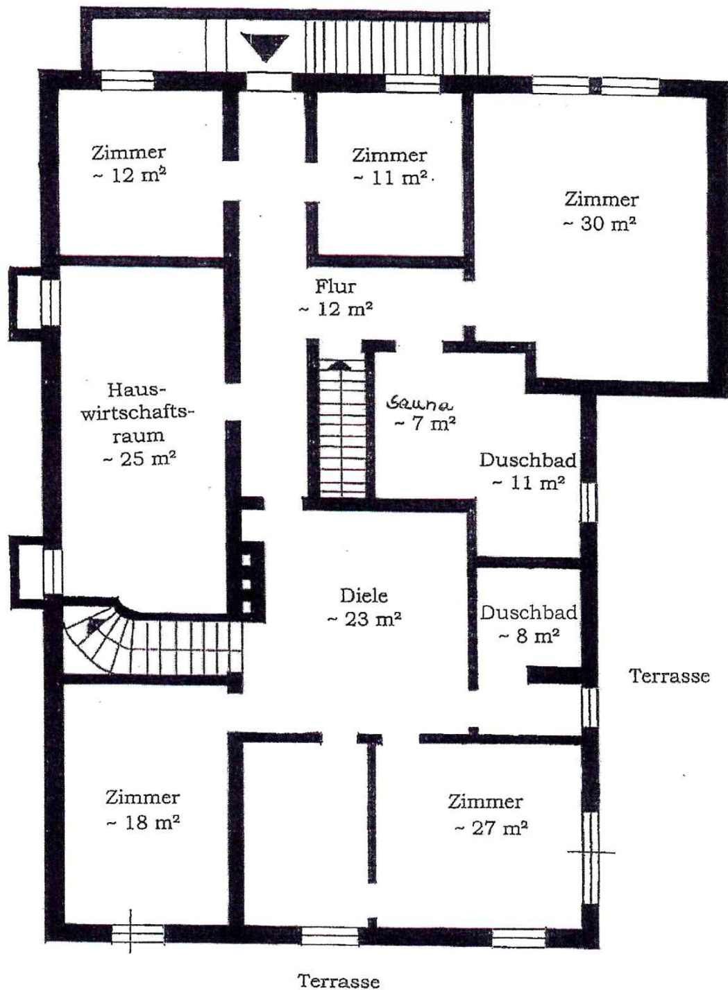
Gartengeschoss Maßstab 1 : 100
