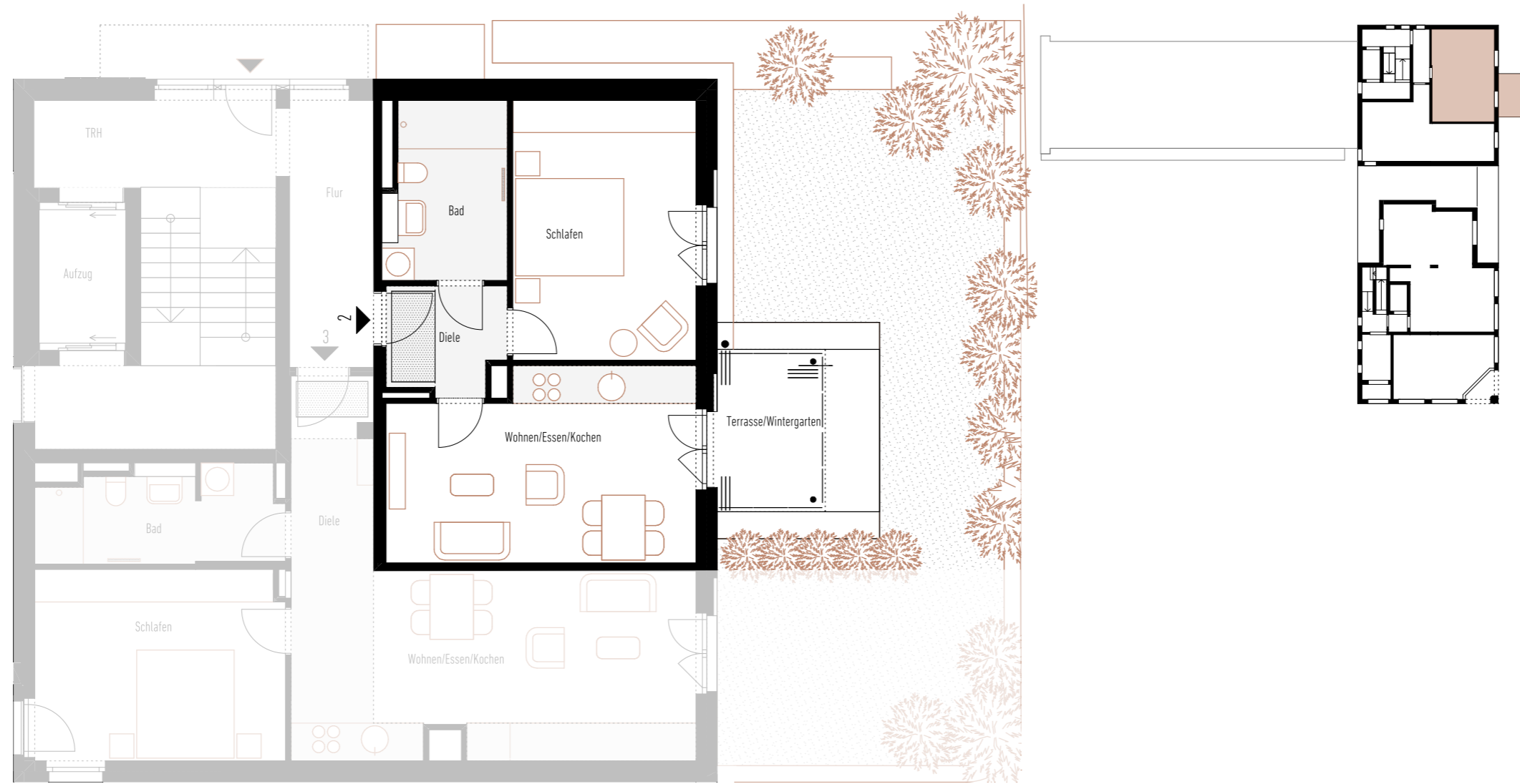
Grundriss Erdgeschoss
