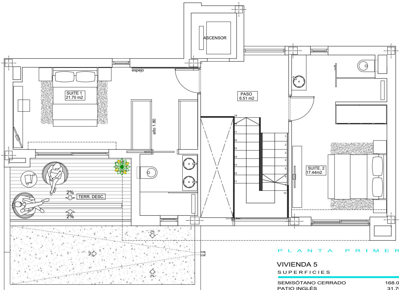
PLANTA PRIMERA
