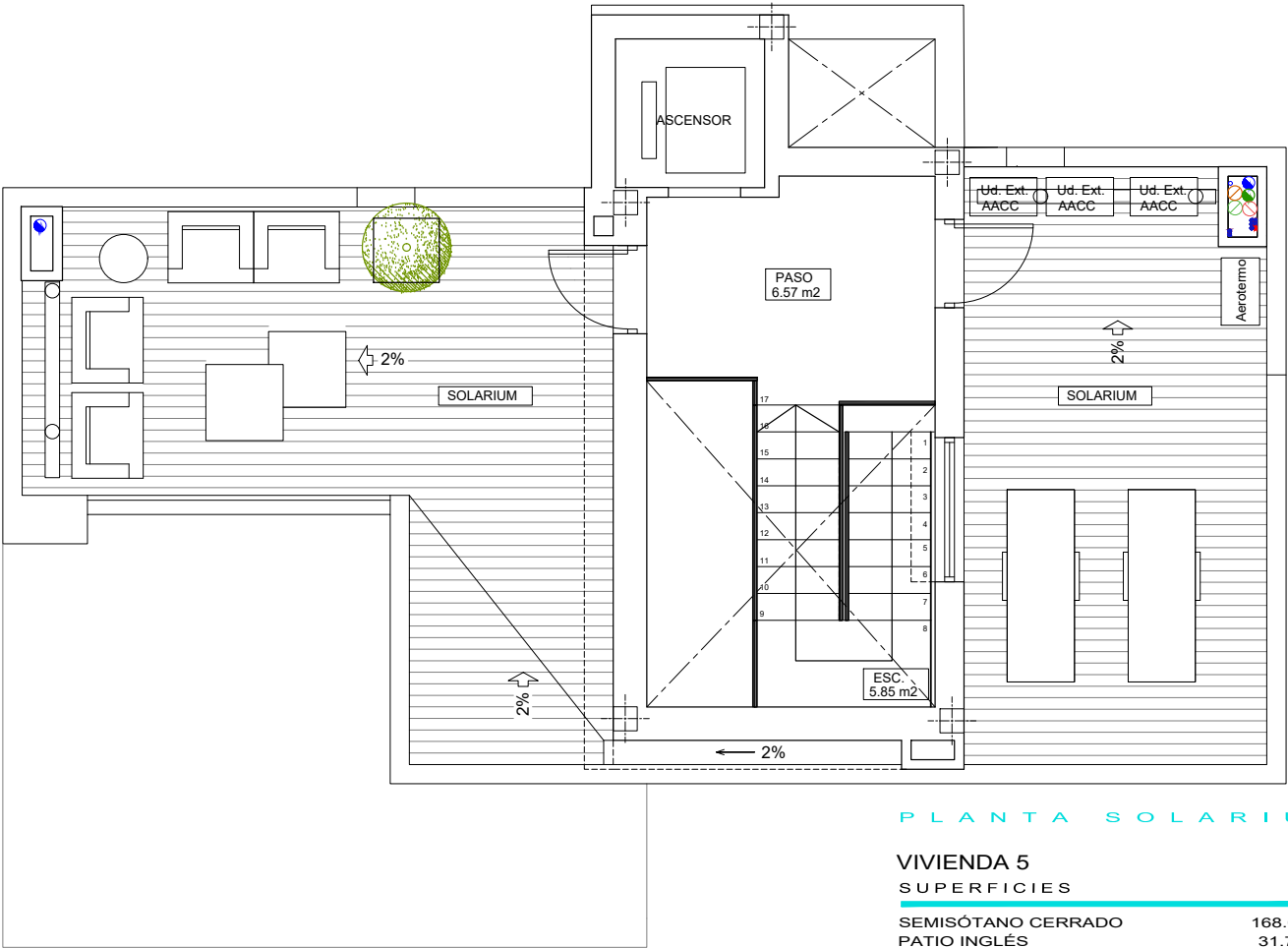
PLANTA SOLARIUM
