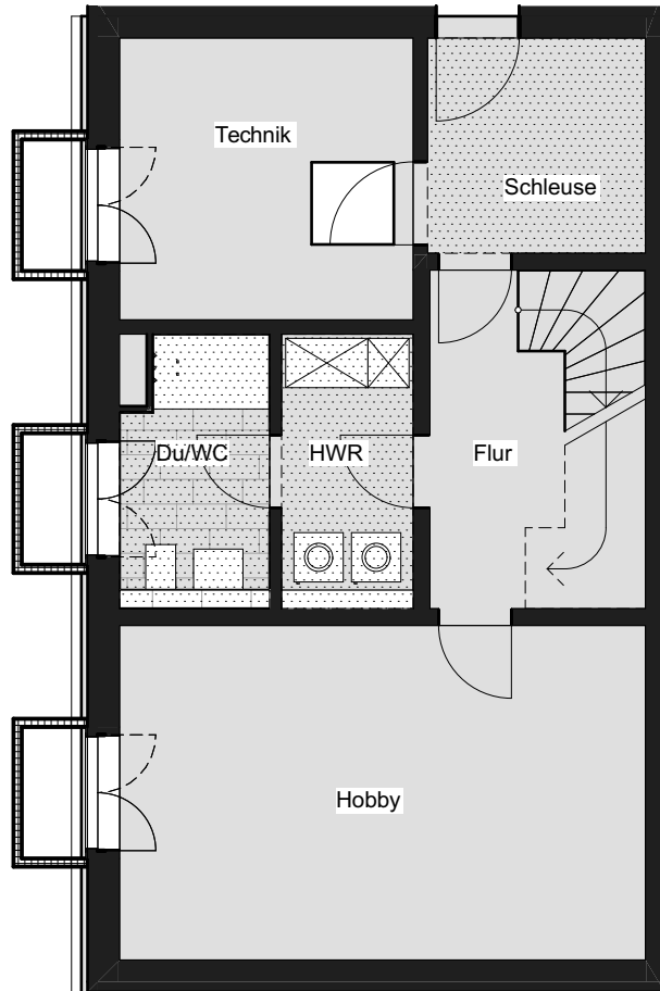
Kellergeschoss DHH 1
