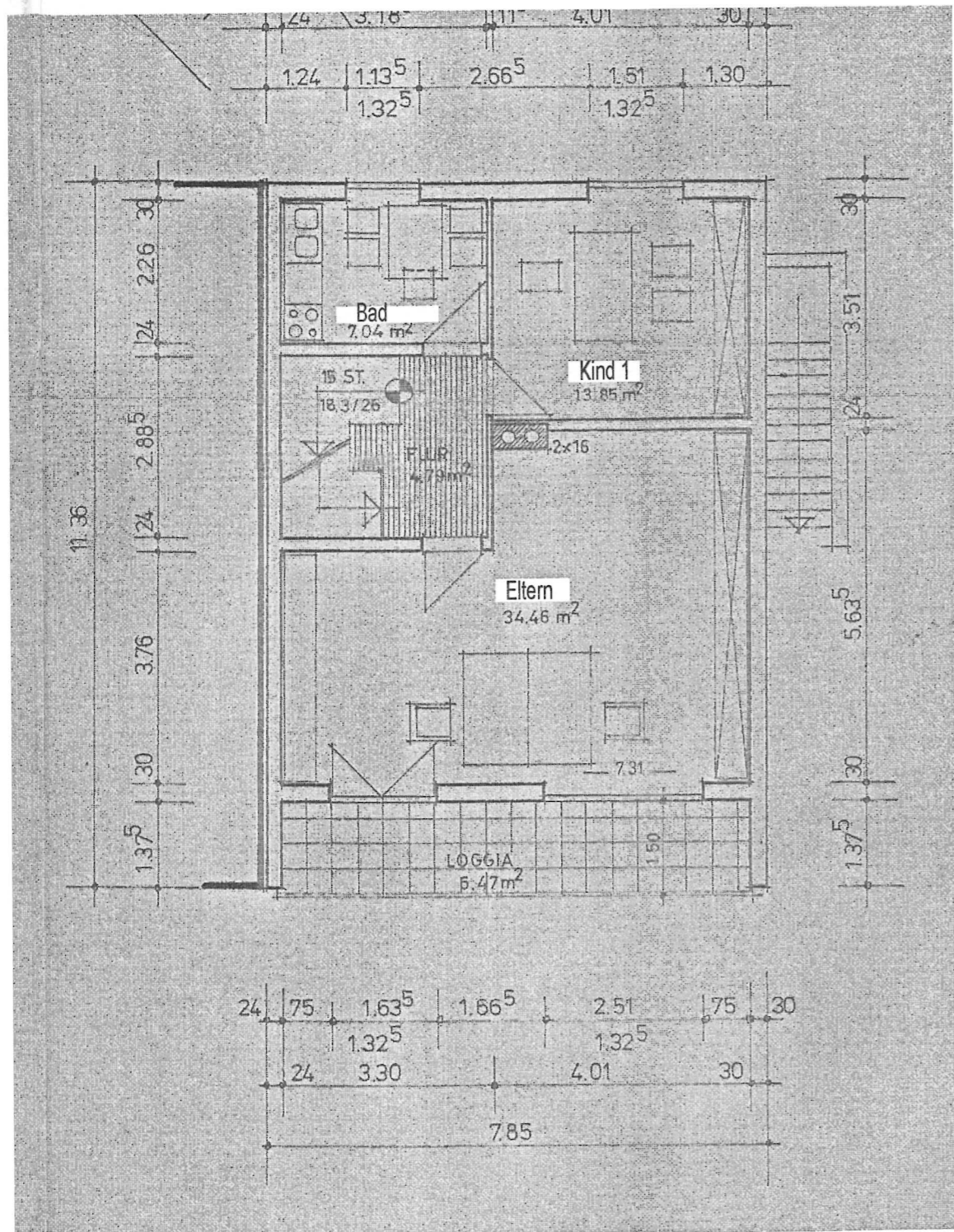
Grundriss Obergeschoss
