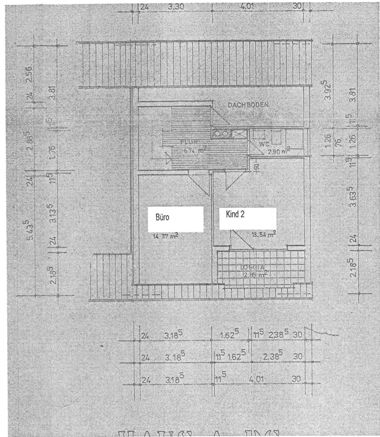
Grundriss Dachgeschoss
