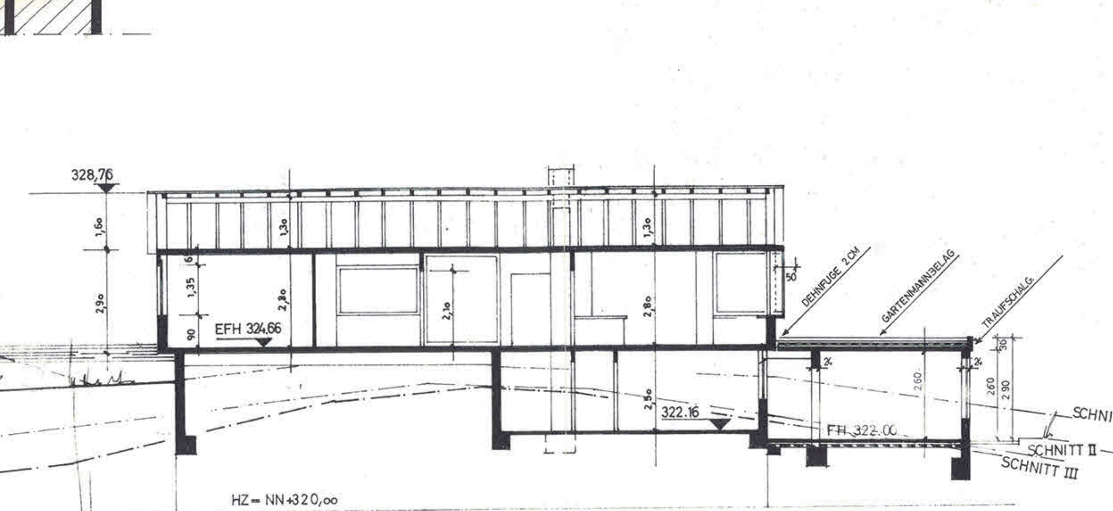
SCHNITT I-I
