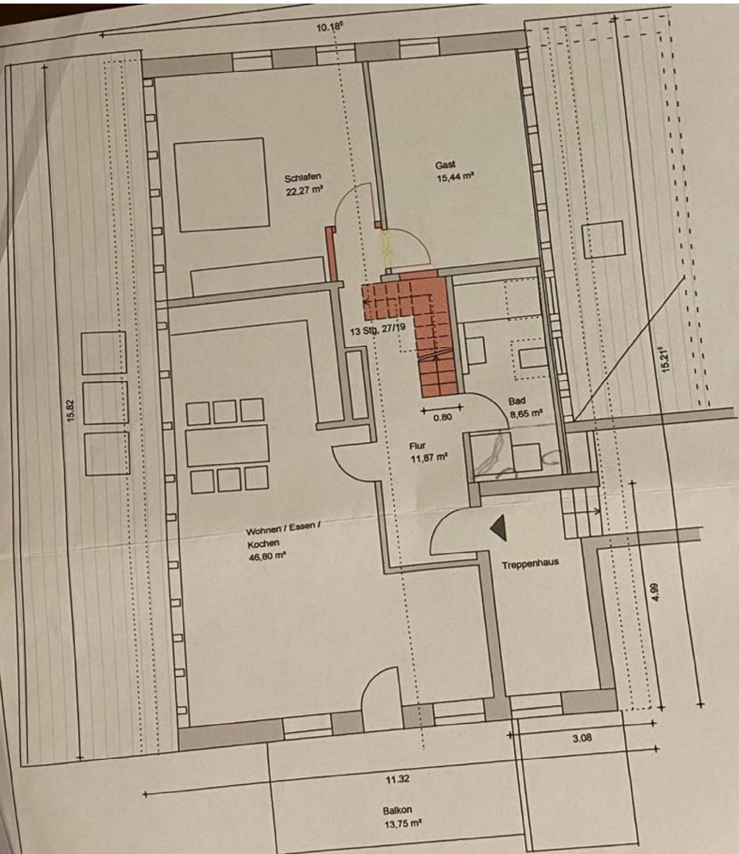
Grundriss 2. DG
