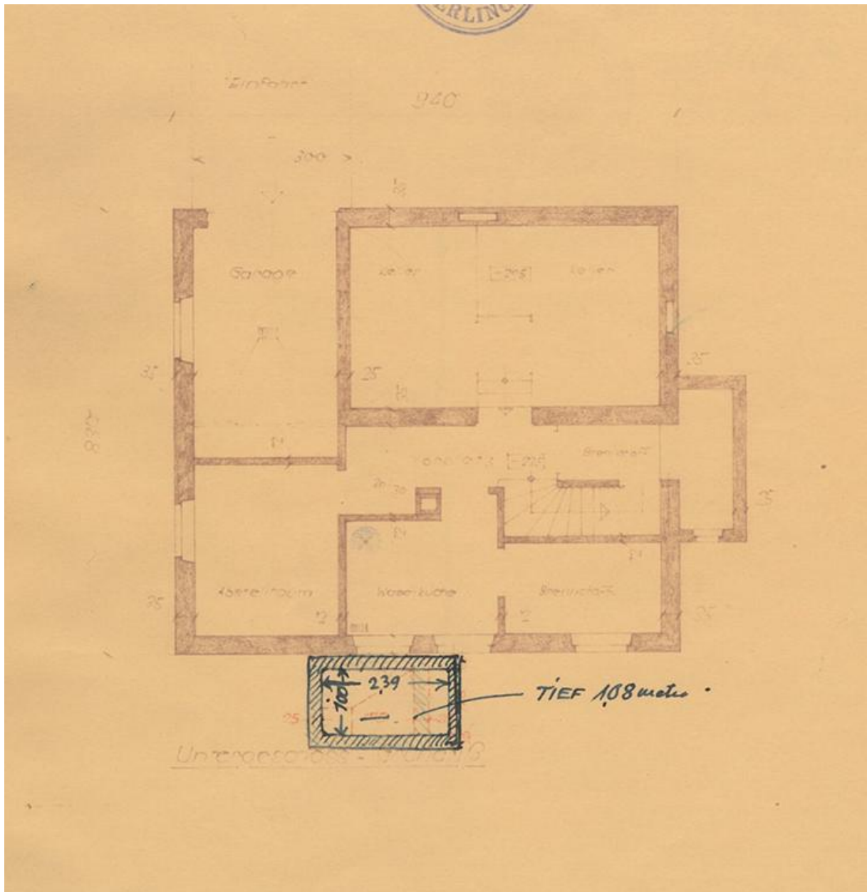
Kellergeschoss
