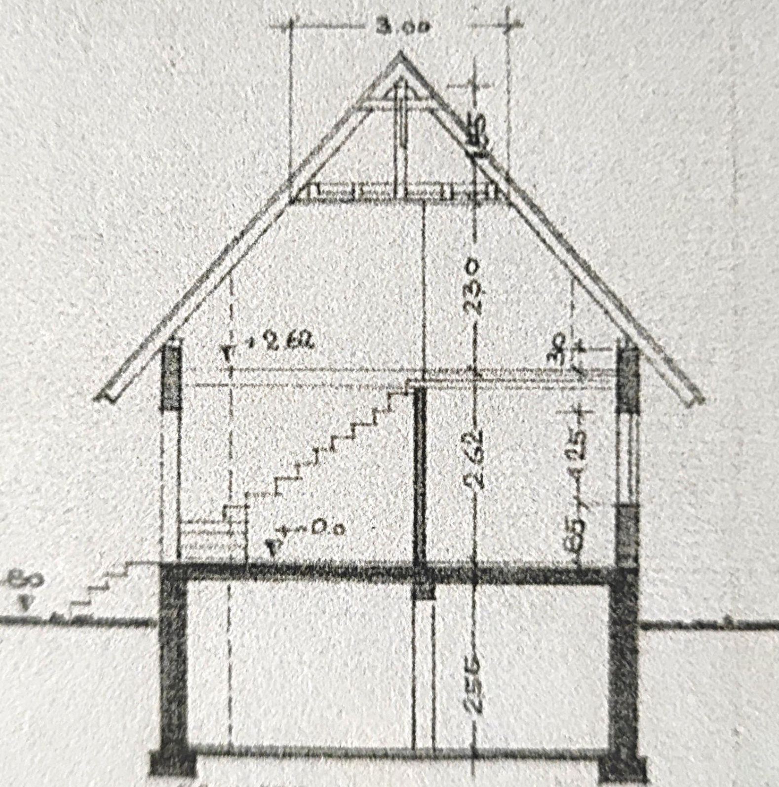
SCHNITT A-B
