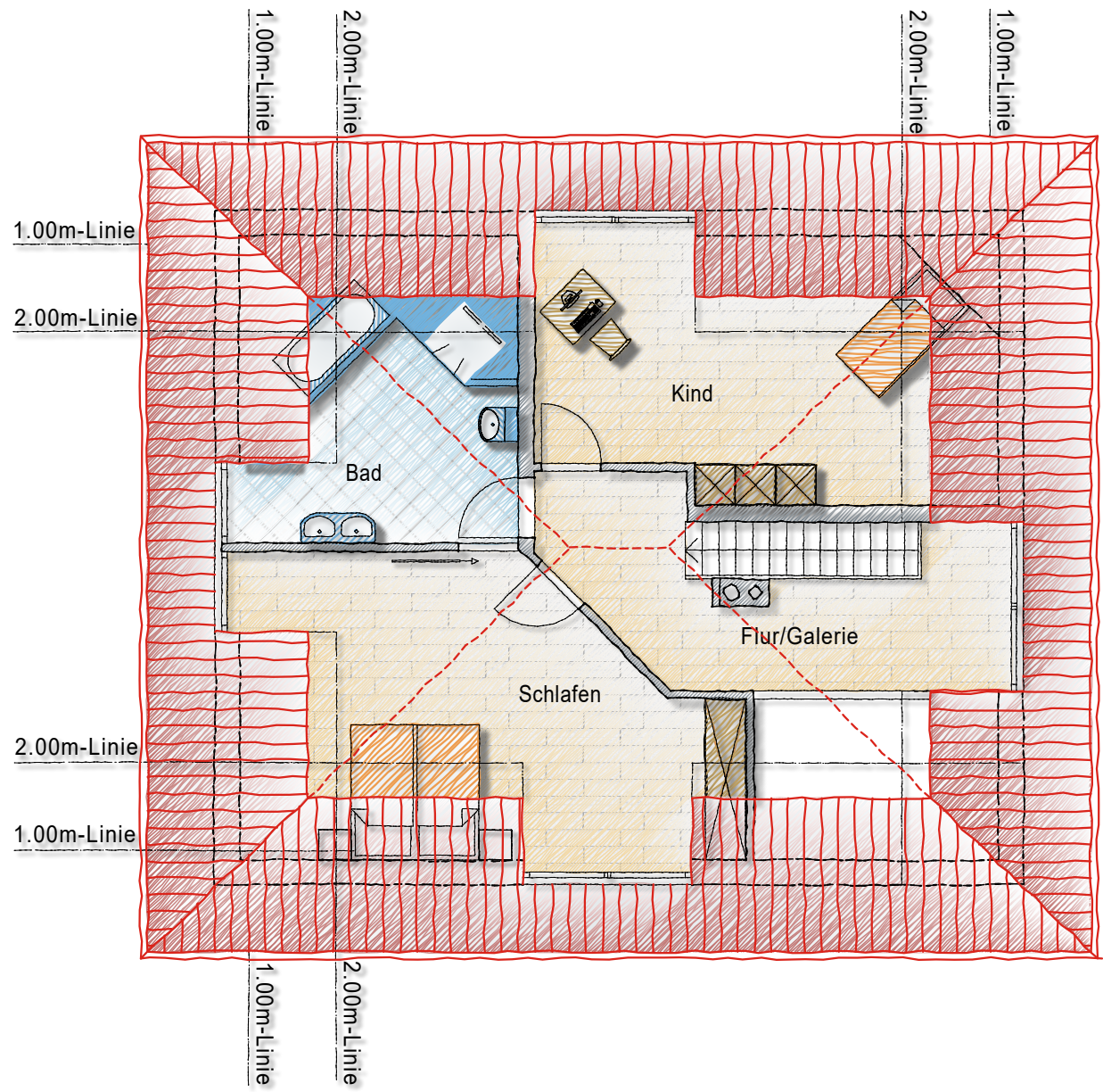
Dachgeschoss
