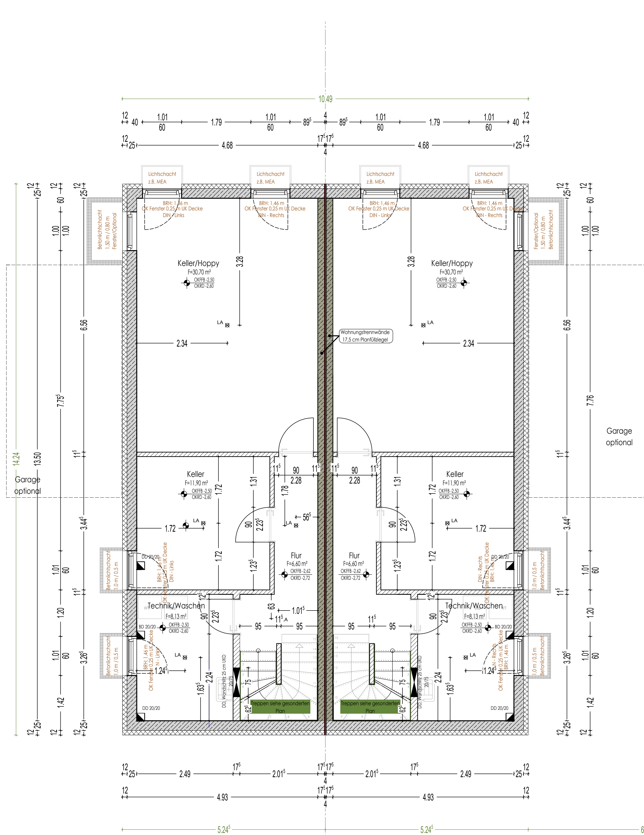
Doppelhaus 1
