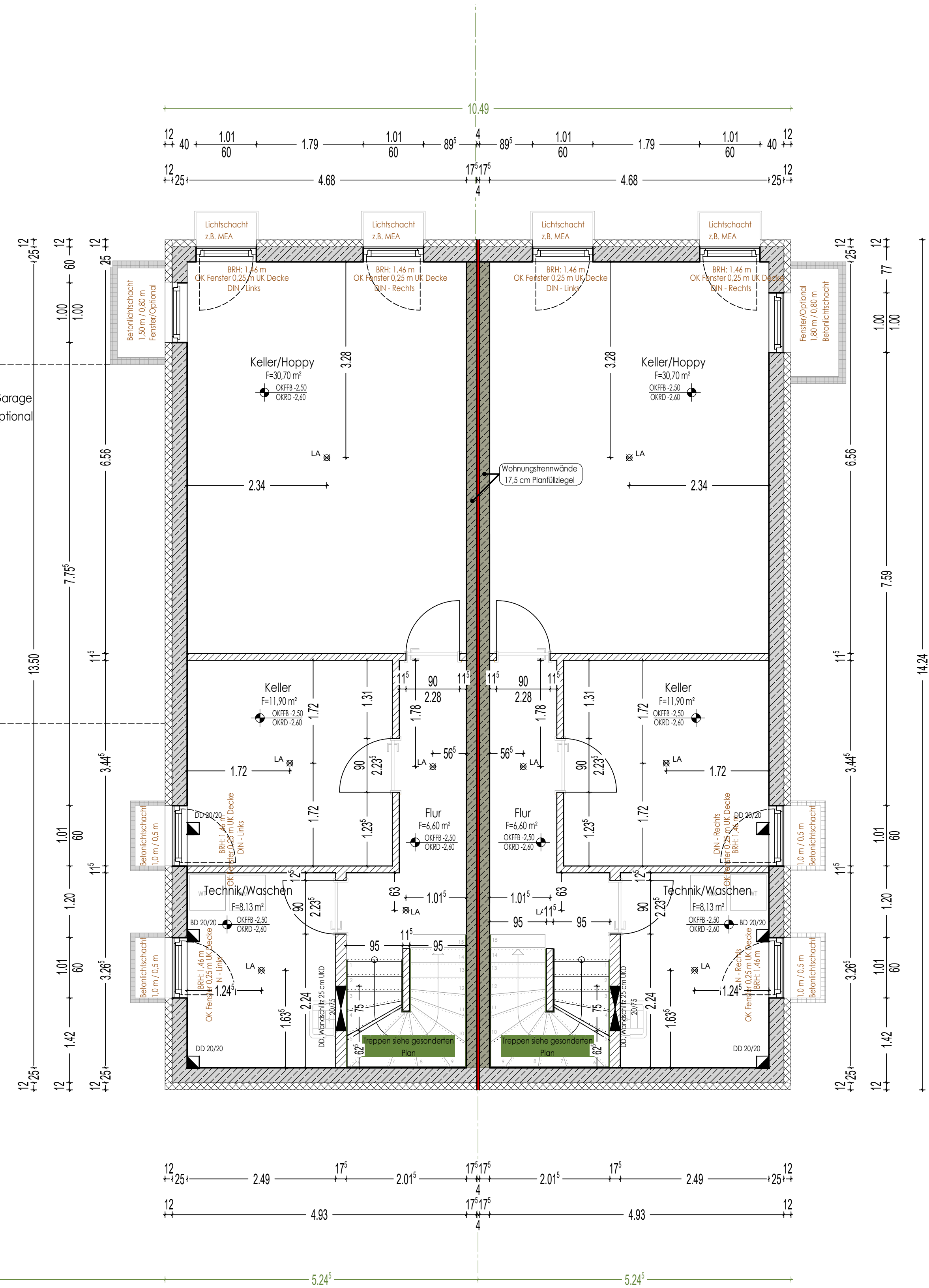
Doppelhaus 2
