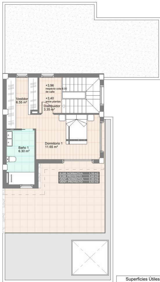
PL. PISO
