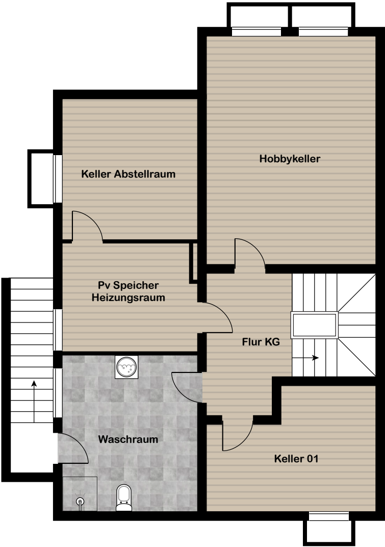
Kellergeschoss
