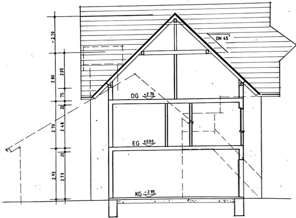
QUERSCHNITT
