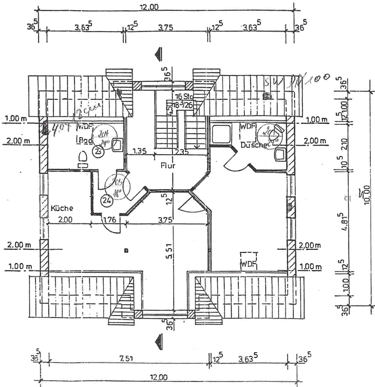
Grundriß DG
