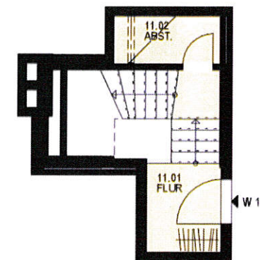
Obergeschoss/ Eingangsbereich
