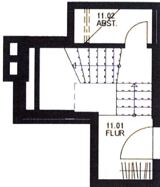
Obergeschoss/ Eingangsbereich
