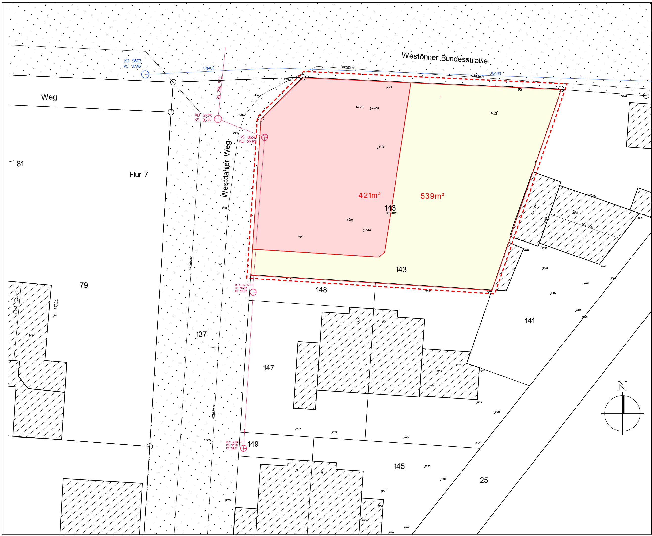
Lageplan Baugrundstücke Westdähler Weg 59457 Werl-Westönnen Westdählerweg 59457 Werl Maßstab 1:250
