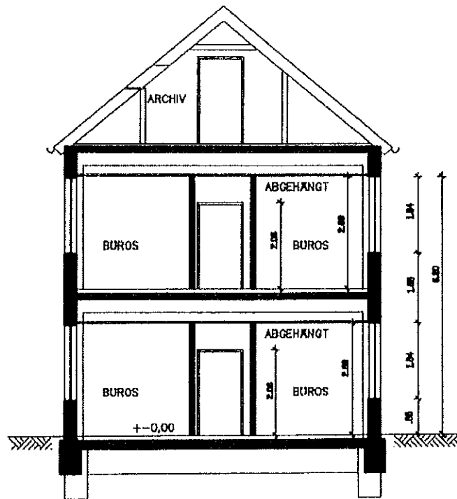
QUERSCHNITT
