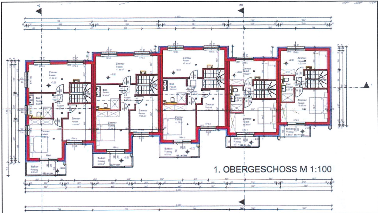
Abbildung 10: Grundrissplan 1. Obergeschoss
