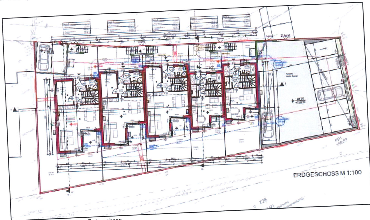
Abbildung 9: Grundrissplan Erdgeschoss
