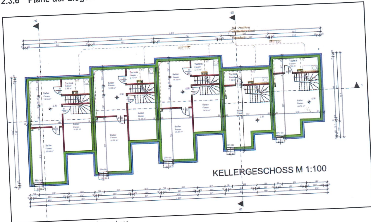
Abbildung 8: Grundrissplan Kellergeschoss
