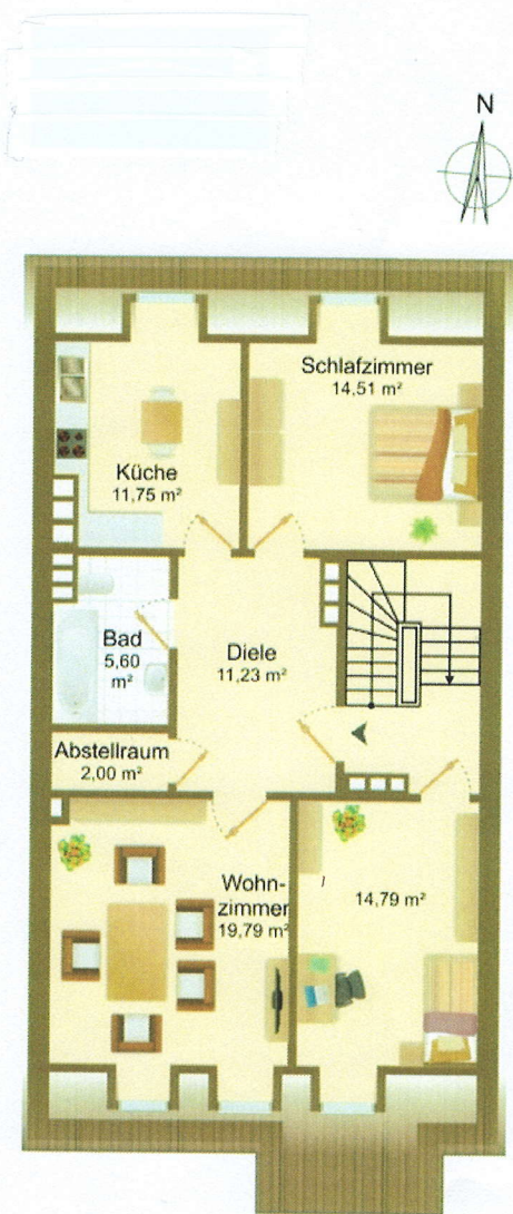
Grundriss DG
