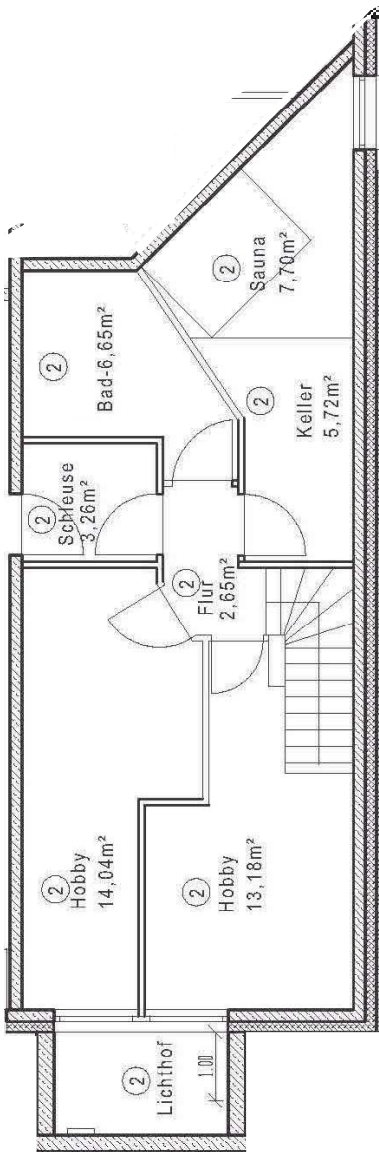
Untergeschoß Hobby: mit eigenem Zugang und 2,90 m hohen Oberlichtern/Fenstern
