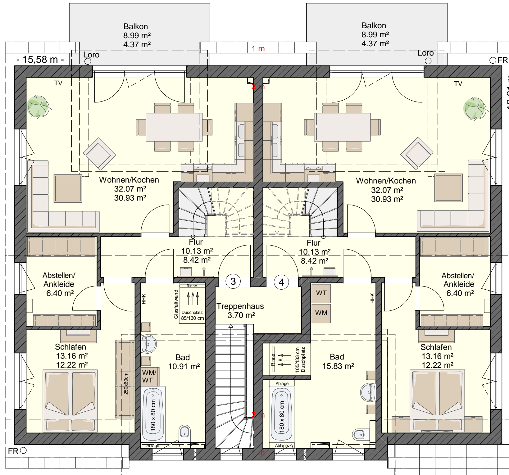
GRUNDRISS DACHGESCHOSS Wohnung 3+4
