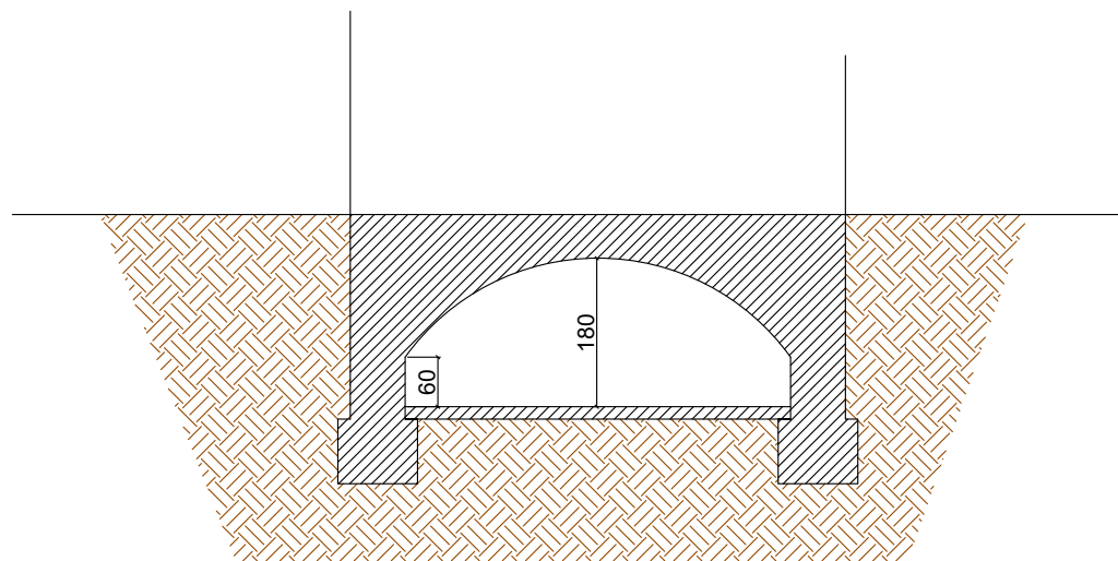
SYSTEMSCHNITT AA
