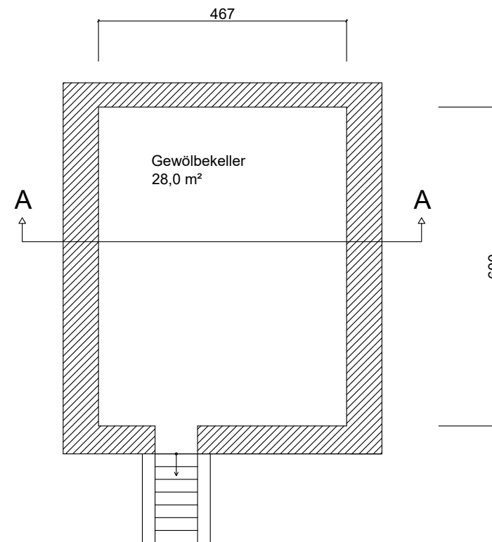
GRUNDRISS KELLERGESCHOSS
