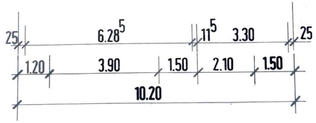
GRUNDRISS DACHGESCHOSS
