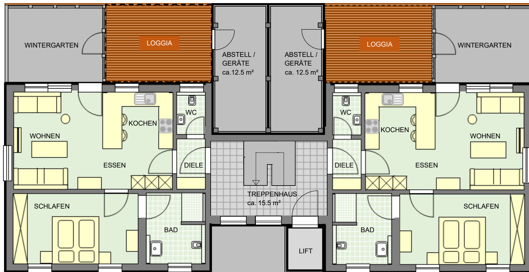
GRUNDRISS OBERGESCHOSS
