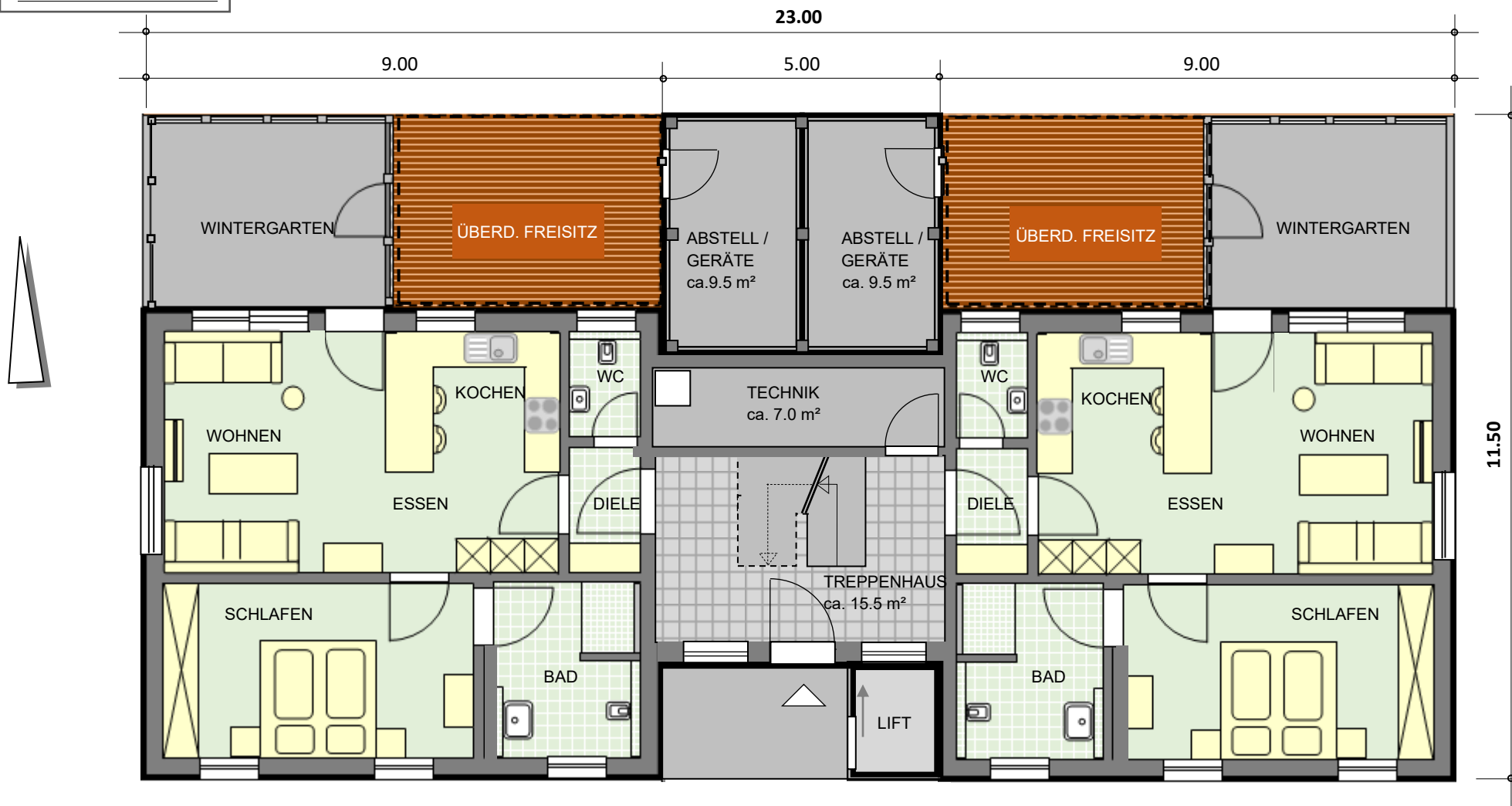
GRUNDRISS ERDGESCHOSS
