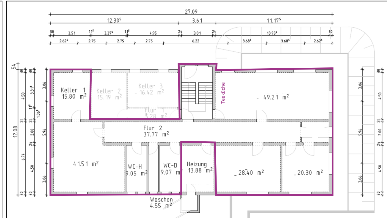
Grundriss Souterrain
