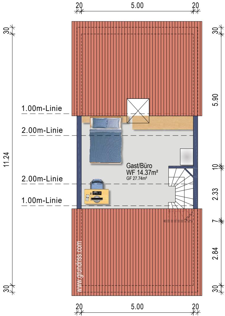
Dachgeschoss
