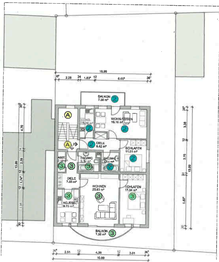
OBERGESCHOSS-GRUNDRISS
