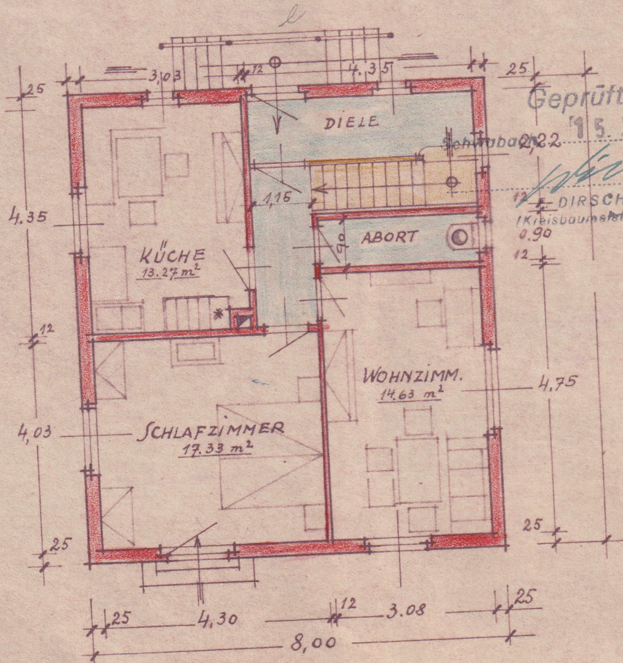
ERDGESCHOSS
