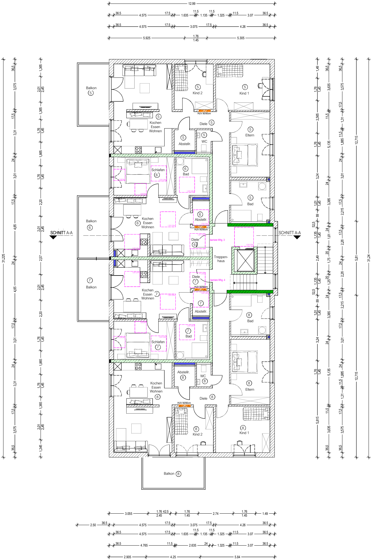
Grundriss 1. Obergeschoss
