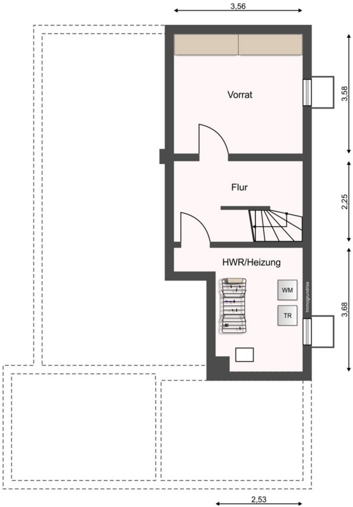
Kellergeschoss
