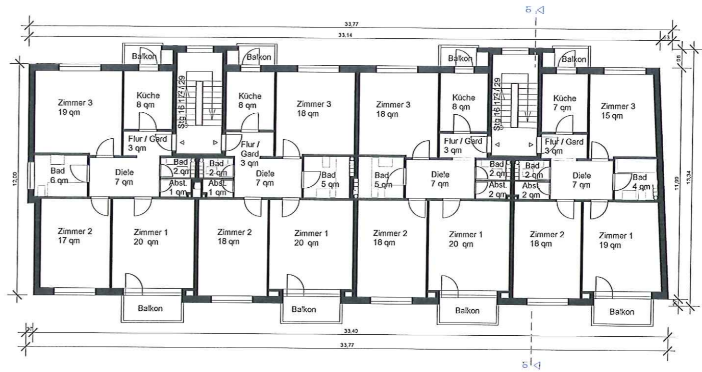
Bestand Grundriss 3.OG
