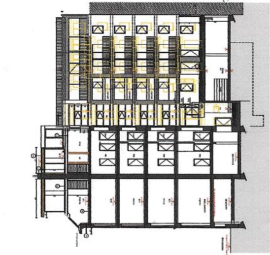
Schnitt B-B 1:100
