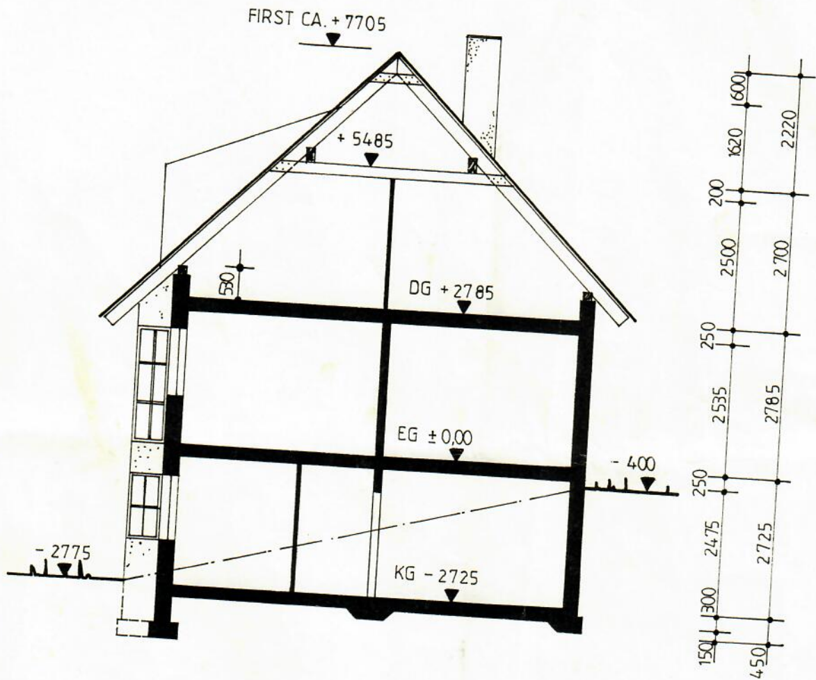
QUERSCHNITT
