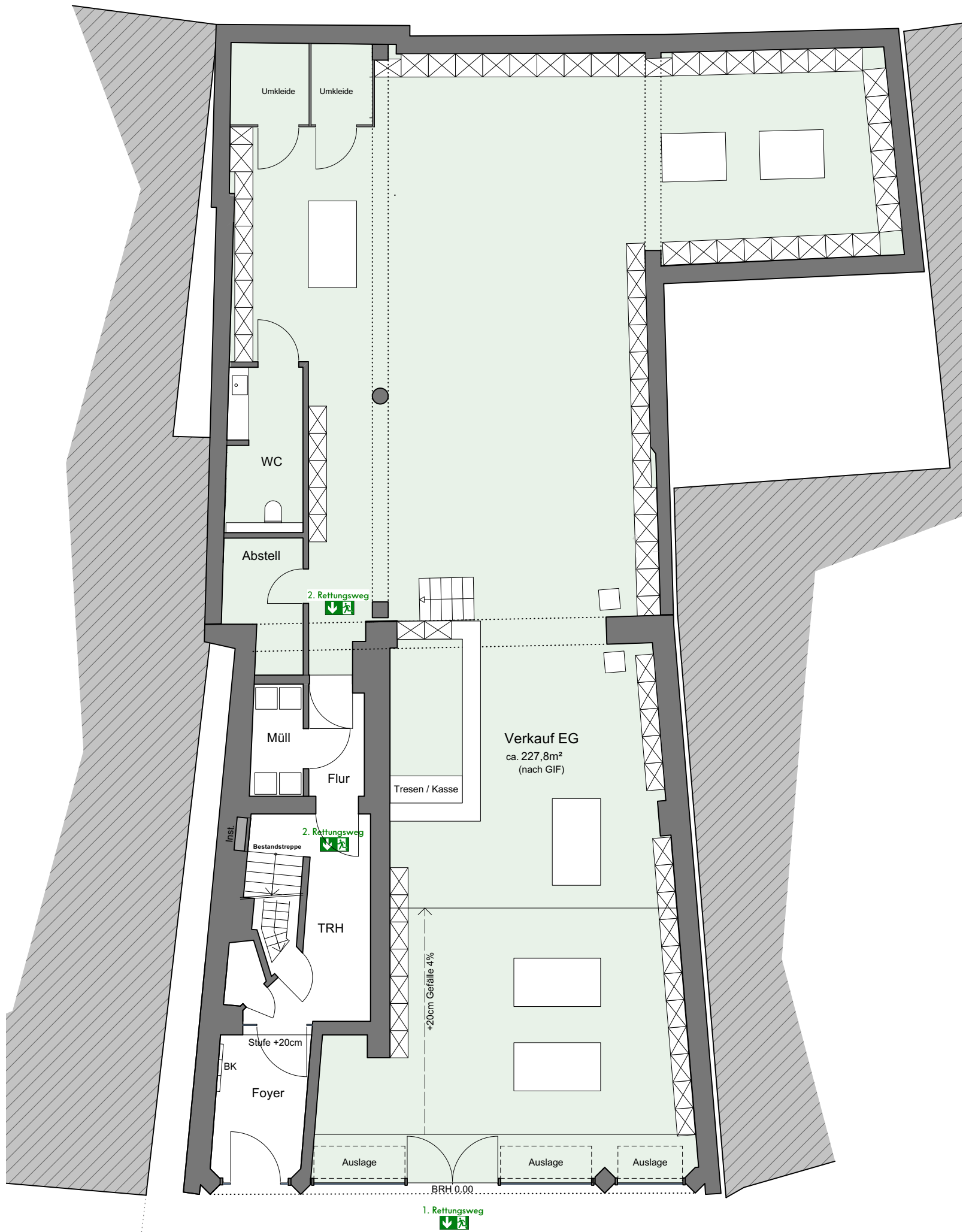
Grundriss EG - Beispielplanung
