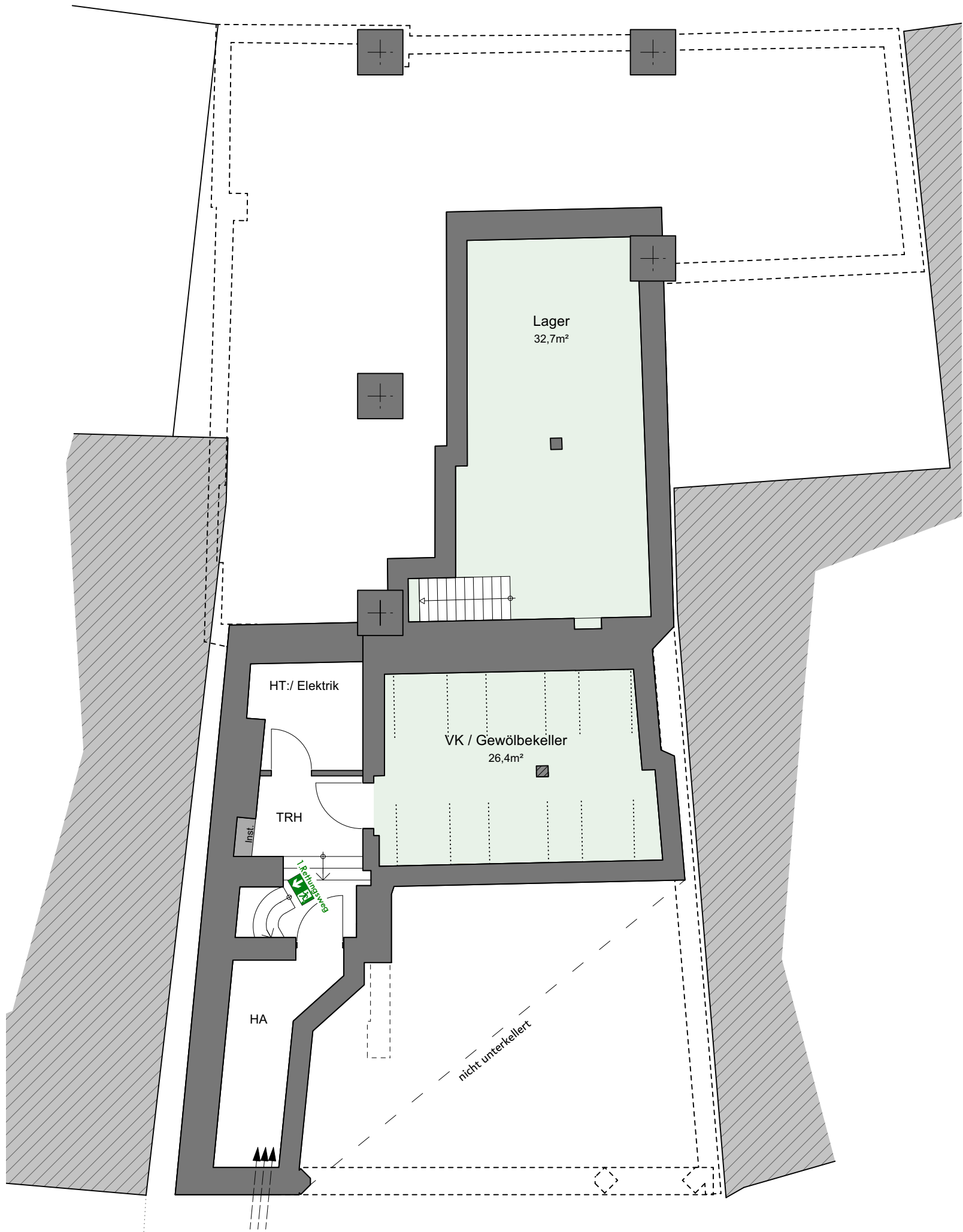
Grundriss KG - Beispielplanung
