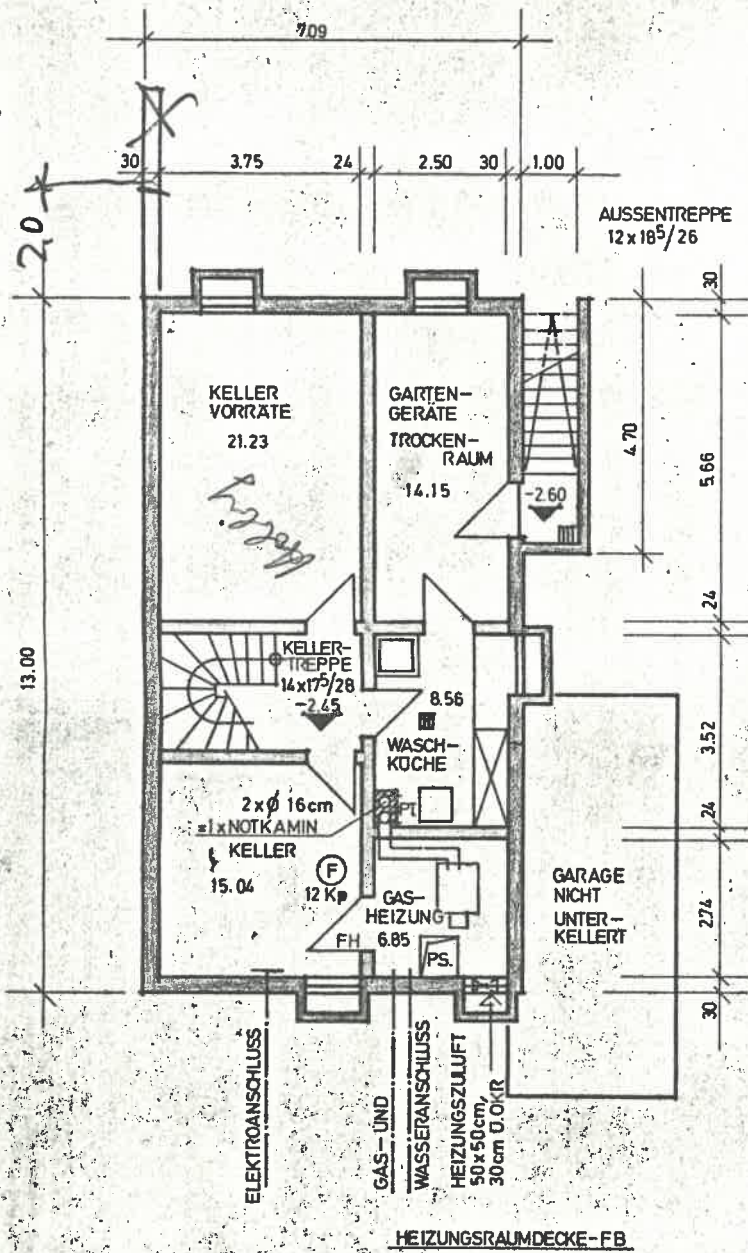
KELLERGESSCHOSS
