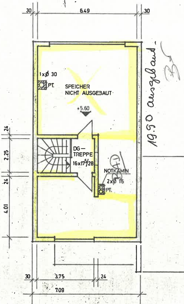
DACHGESCHOSS
