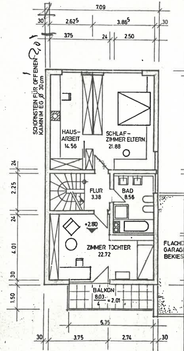
OBERGESCHOSS
