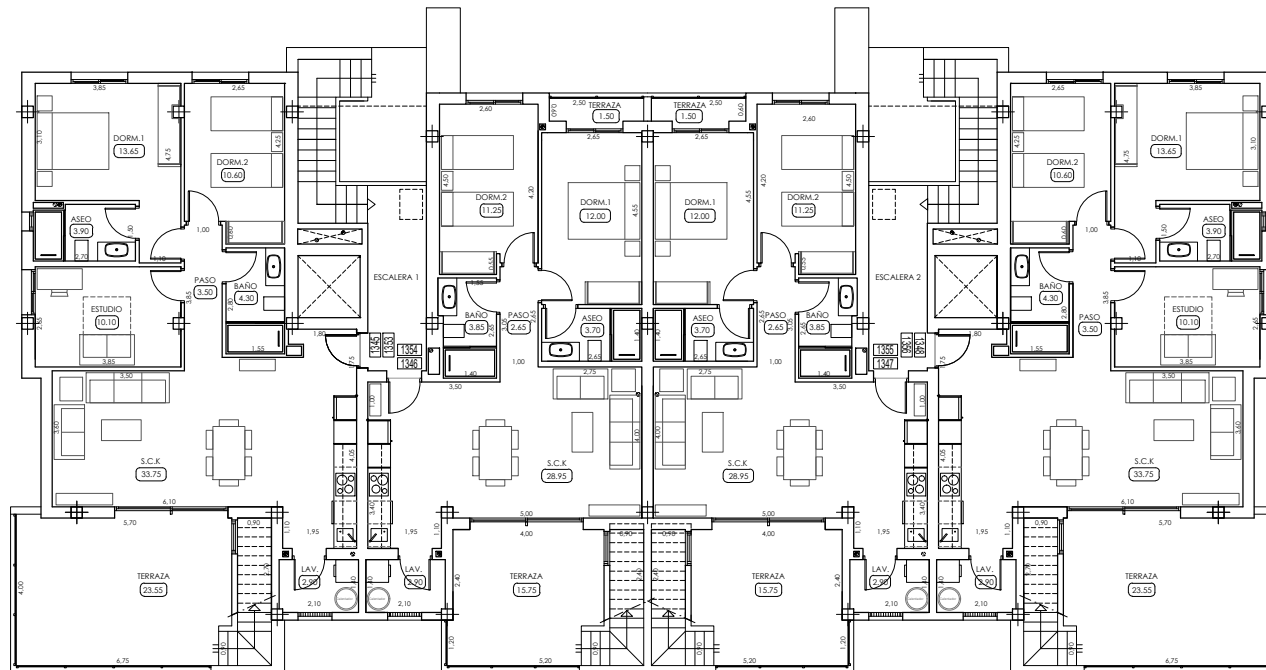
PL PRIMERA
