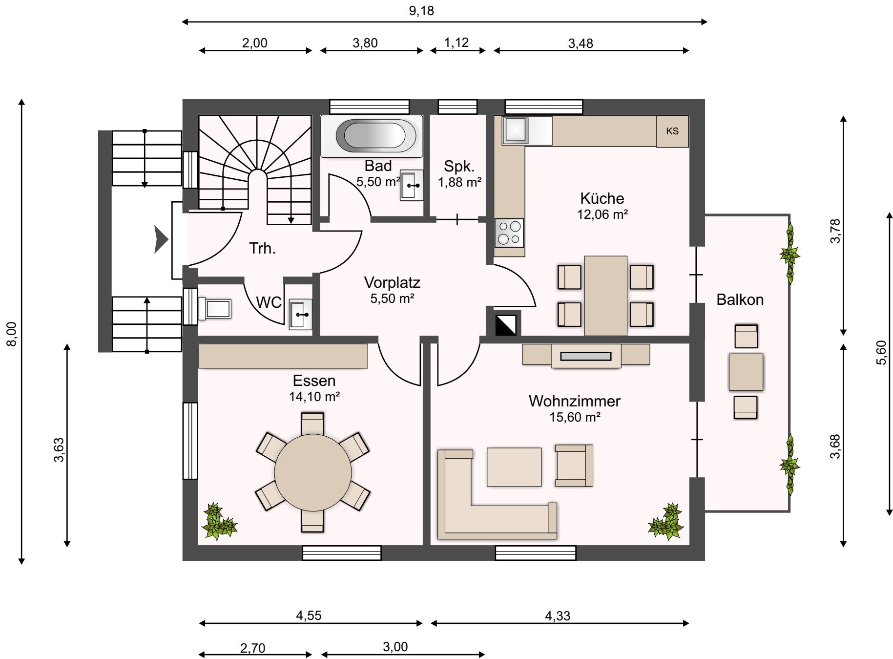
Erdgeschoss
