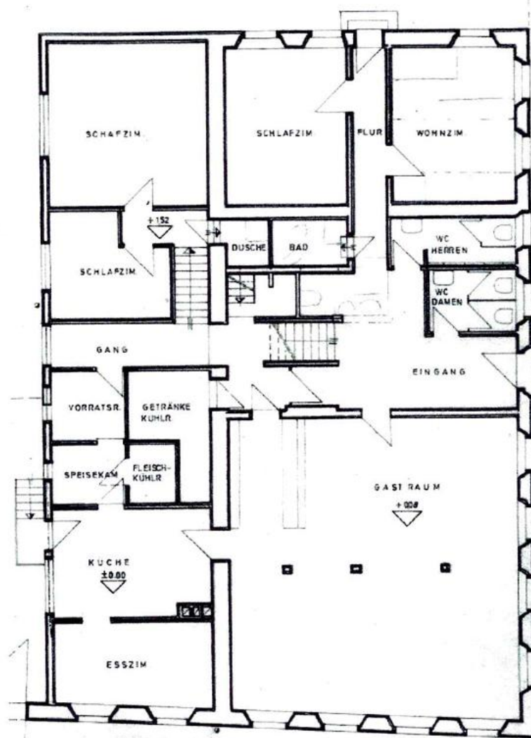
Erdgeschoss
