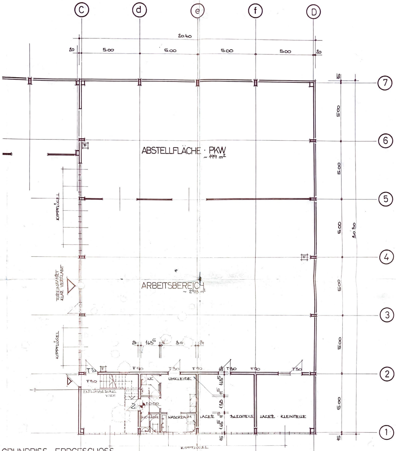
GRUNDRISS · ERDGESCHOSS
