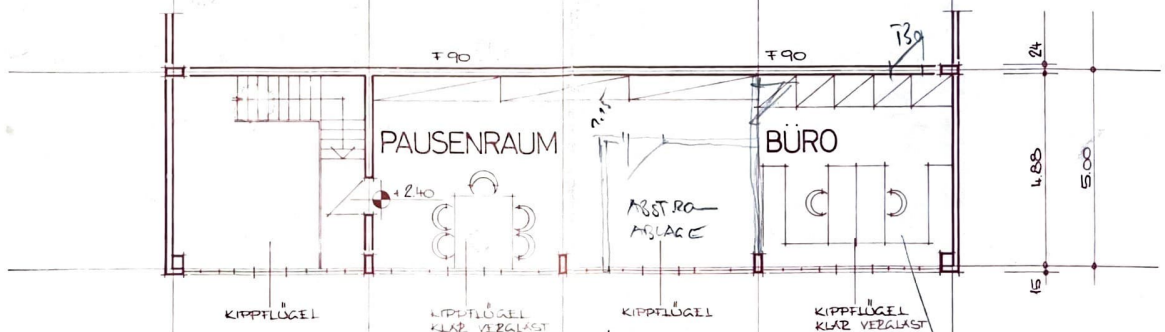
GRUNDRISS · ERDGESCHOSS
